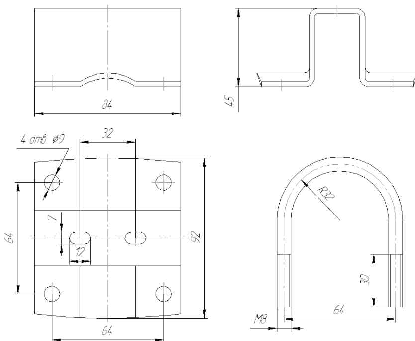
Рис. 4-2. Кронштейн Т, скоба для блока клапанного С30, (БКНЗ).
