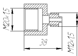
Рис. 4-12. Переходник ПР M12.
