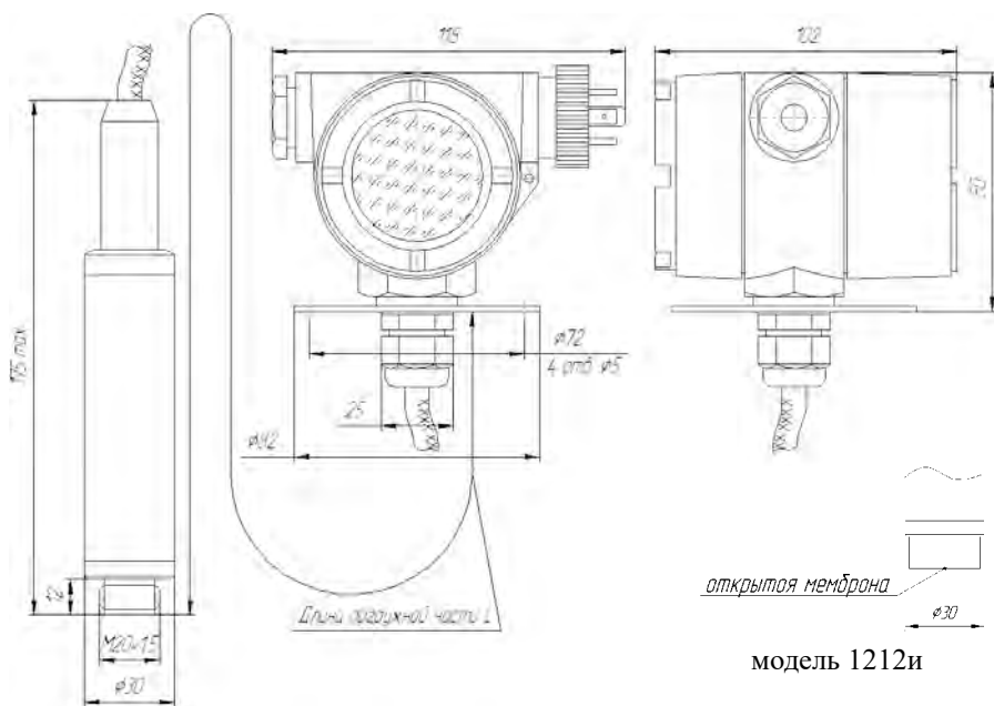
Модель 1210, 1212. Индикация.
