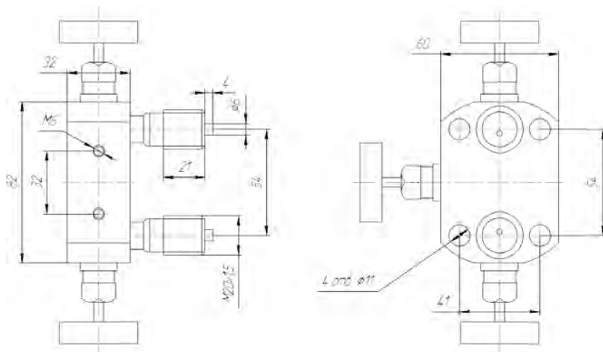
Рис. 4-1. Блок клапанный С 30 (БКН 3-11).
