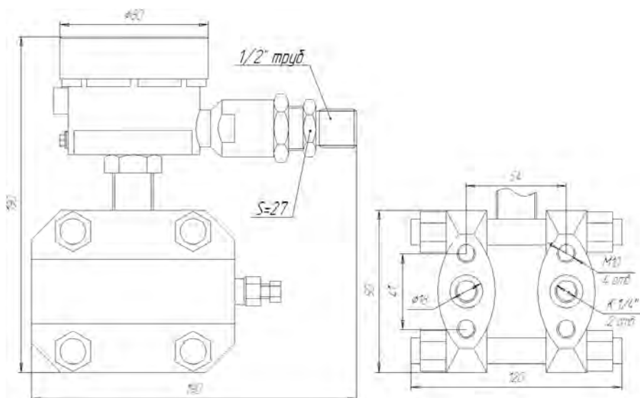
Рис. 3-17. Модель 1167. Взрывонепроницаемая оболочка , стальной корпус, ввод под трубу или бронированный кабель.
