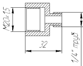
Рис. 4-11. Переходник ПР 1/4.
