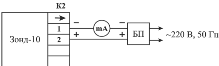
Рис.2-2. Подключение датчиков для соединения K2 в режиме выходного сигнала 4 \div 20\text{мА} *.
