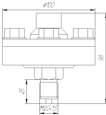
Рис. 4-22. Разделительная мембрана РМ5321
