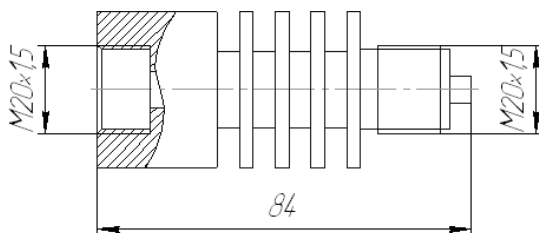
Рис. 4-14. Штуцер термобагающий. До 150°C (При горизонтальной установке).
