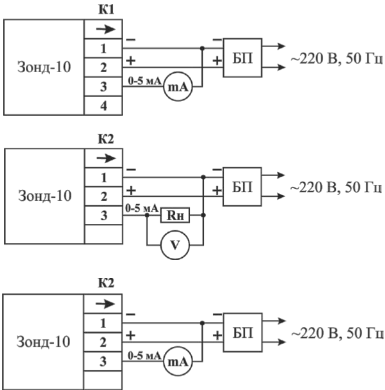
Рис.2-3. Подключение датчиков для соединения K1, K2 в режиме выходного сигнала 0 \div 5\text{ мА} .
