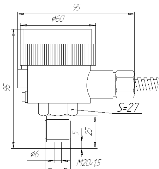
Рис. 3-08. Модель 1190, 1200 Взрывонепроницаемая оболочка, нержавеющей корпус, встроенный кабель.
