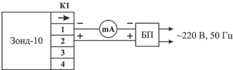
Рис.2-1. Подключение датчиков для соединения K1 в режиме выходного сигнала 4 \div 20\text{мА} *.
