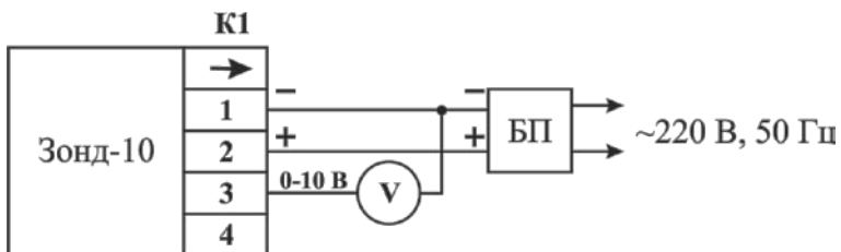
Рис.2-4. Подключение датчиков для соединения K1 в режиме выходного сигнала 0 \div 10\text{ В} .
