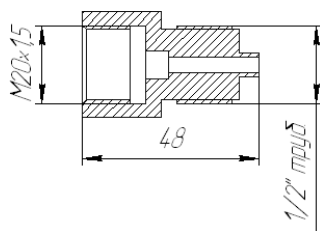
Рис. 4-10. Переходник ПР 1/2.
