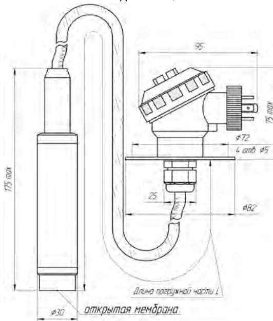
Модель 1212.
