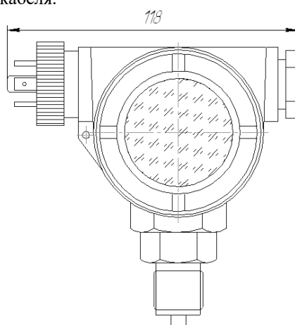
Гермоввод кабеля.
