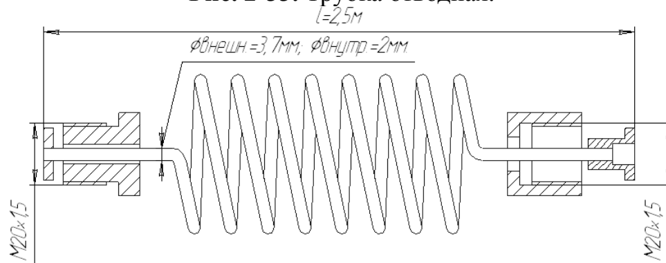
Рис. 2-34. Трубка импульсная.
