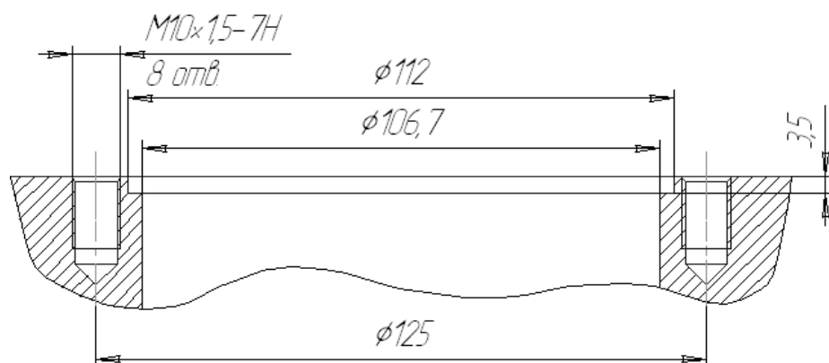
Рис. 2-36. Место установки разделителя РМ5320
