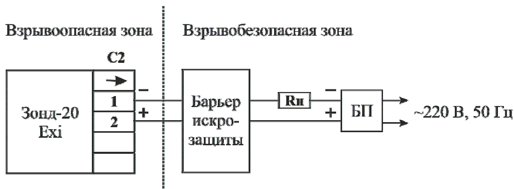
Рис.7. Подключение датчиков для соединения С2 в режиме выходного сигнала 4 \div 20 мА для Exi исполнения.
