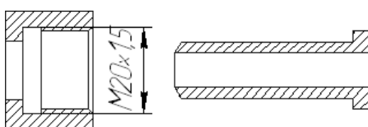
Рис. 2-26. Гайка, ниппель.
