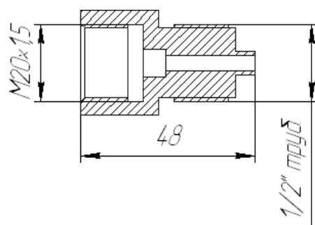
Рис. 2-28. Переходник ПР 1/2.
