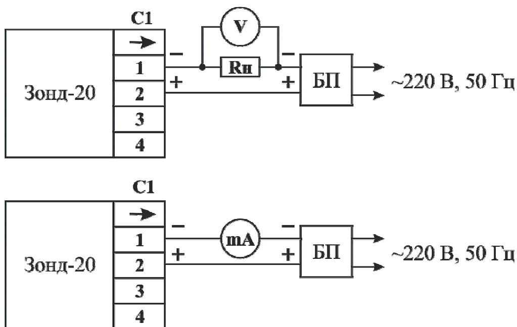
Рис.1. Подключение датчиков для соединения C1 в режиме выходного сигнала 4 ÷ 20мА.
