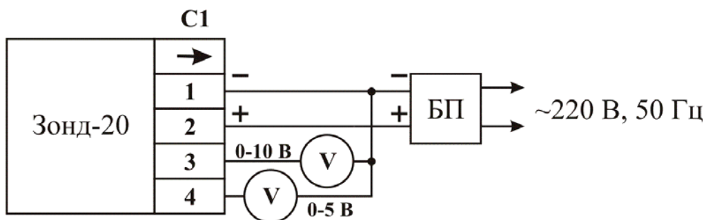
Рис.4. Подключение датчиков для соединения С1 в режиме выходного сигнала 0 \div 10\text{В} , 0 \div 5\text{В} для модели ЗОНД-20-ДД К7И.
