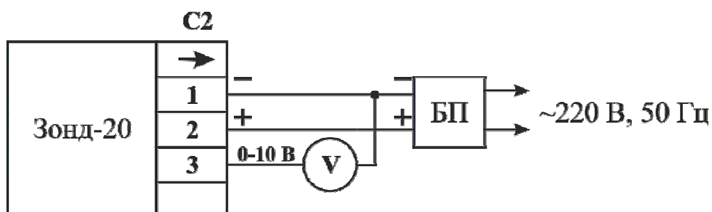
Рис.5. Подключение датчиков для соединения С2 в режиме выходного сигнала 0 \div 10\text{В} .
