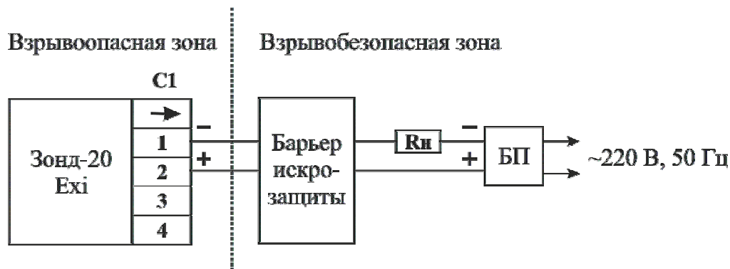
Рис.6. Подключение датчиков для соединения С1 в режиме выходного сигнала 4 \div 20 мА для Exi исполнения.
