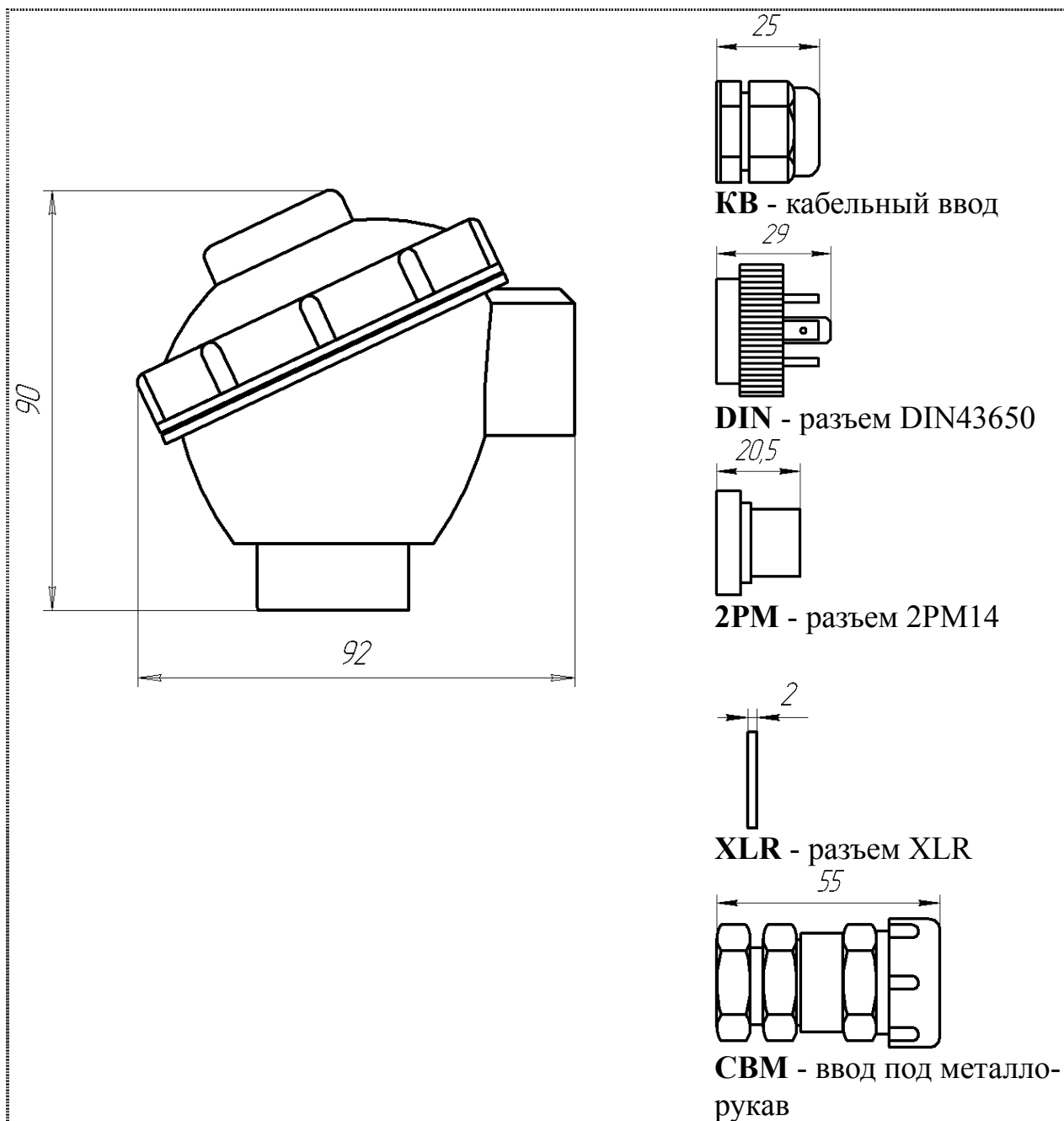
Рис. 2-6. Модель К6
