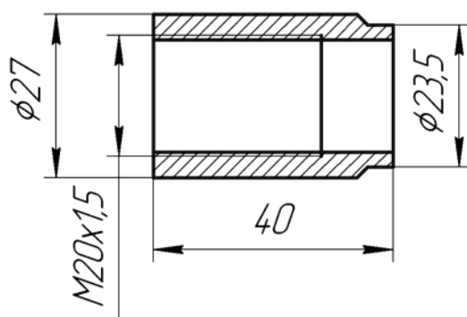
Рис. 2-41. Бобышка вварная
